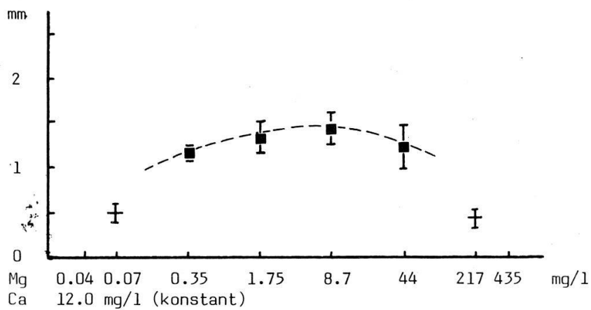
Abb. 5e. Lemna gibba . Mittlere Glieddicken bei verschiedenen Ca- und Mg-Konzentrationen. Abgestorbene Kulturen (†).
