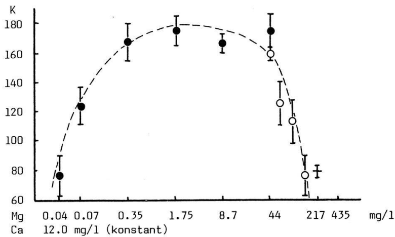
Abb. 2b. Lemna minuscula . Mittlere Wachstumsraten mit Angabe der Standardabweichungen bei verschiedenen Ca- und Mg-Konzentrationen. Ergänzungswerte (O), abgestorbene Kulturen (+).
