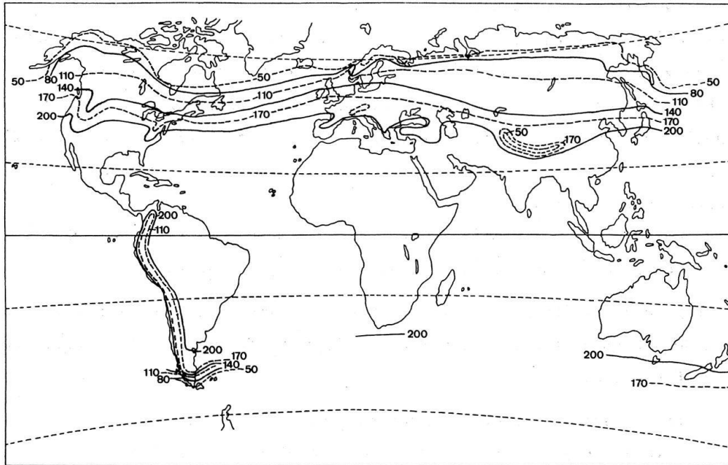
Fig. 1. Number of days with a mean temperature above 10^{\circ}\text{C} Anzahl Tage mit Mitteltemperaturen über 10^{\circ}\text{C}
