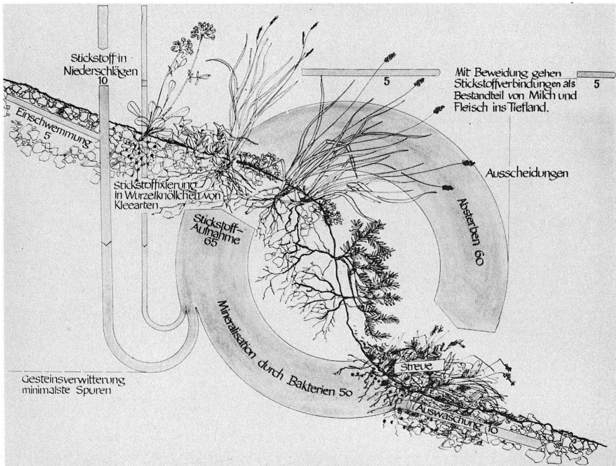
Abb. 1. Stickstoffhaushalt einer subalpinen Blaugrashalde ( Seslerietum ); alle Angaben in kg N/ha/Jahr. Angaben aus REHDER (1970) und Hydrolog. Jahrb. Schweiz (1979), so ergänzt, dass ein Fließgleichgewicht besteht.
