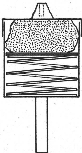
Abbildung 1. Gefriertrommel des Mikrotoms. Trockeneis punktiert. Auf dem Deckel die eingefrorene Wurzel.
