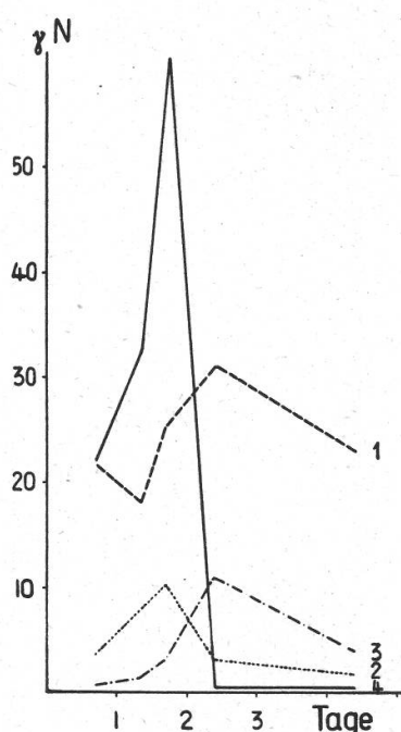
Figur 5 Stickstoffgehalt pro cm 3 Blutungssaft. (Tabelle 10.)
