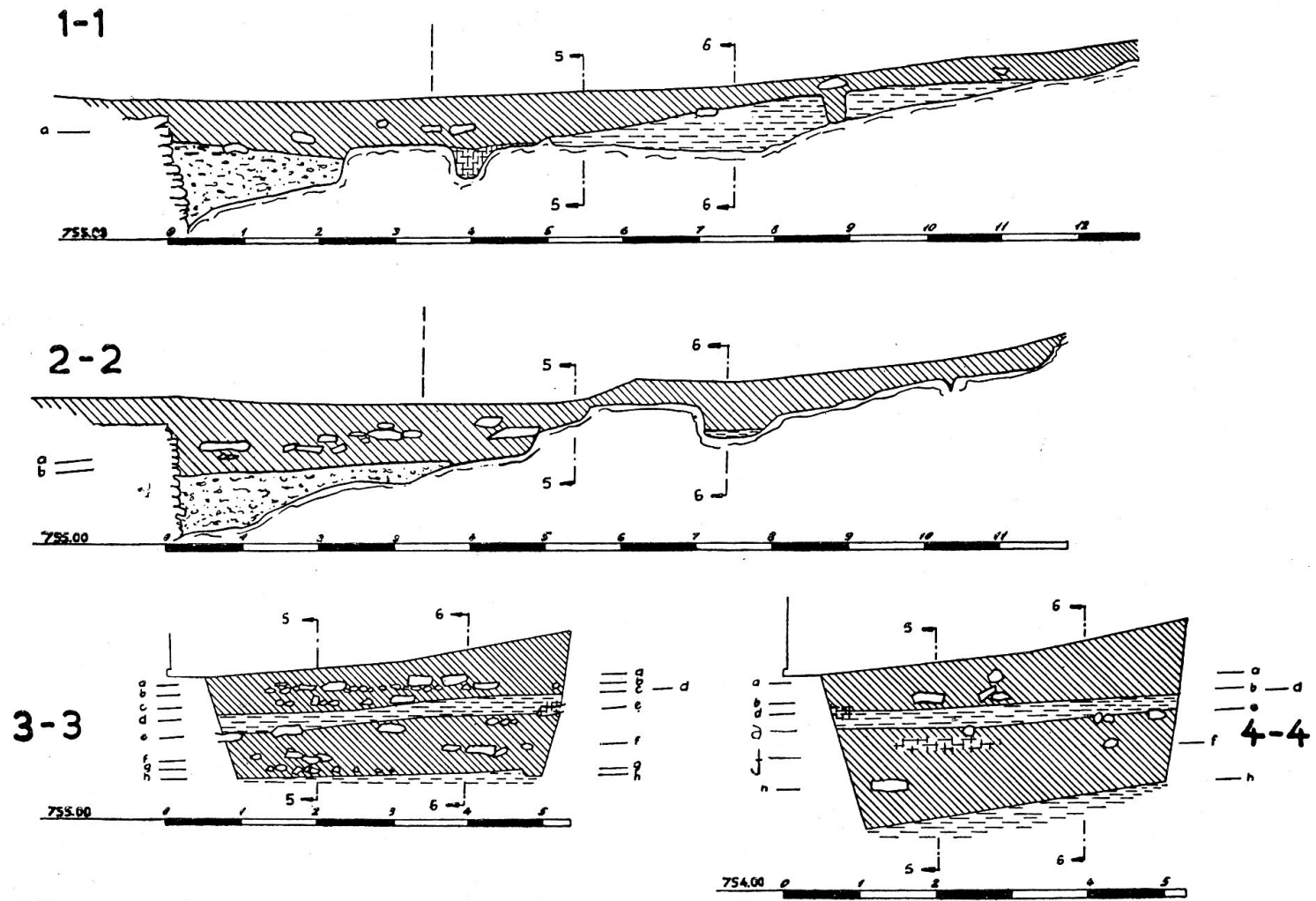
Beil. VIII: Längenprofile
