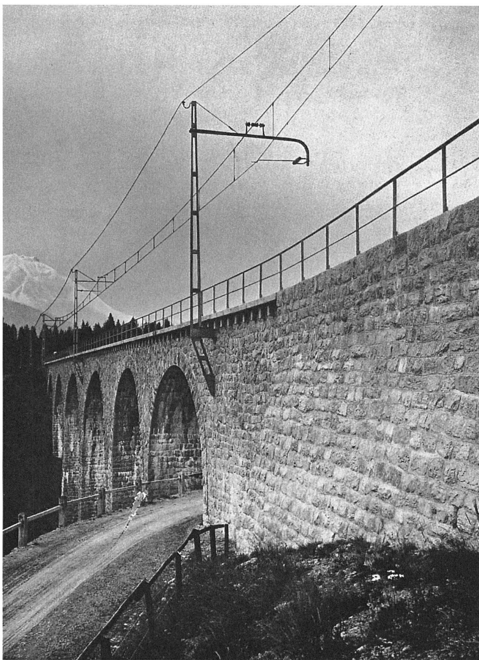
Val-Susauna-Viadukt 1913
