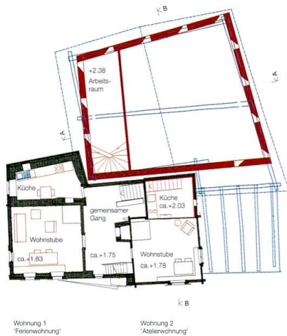
1.Obergeschoss
