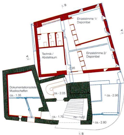
Untergeschoss
