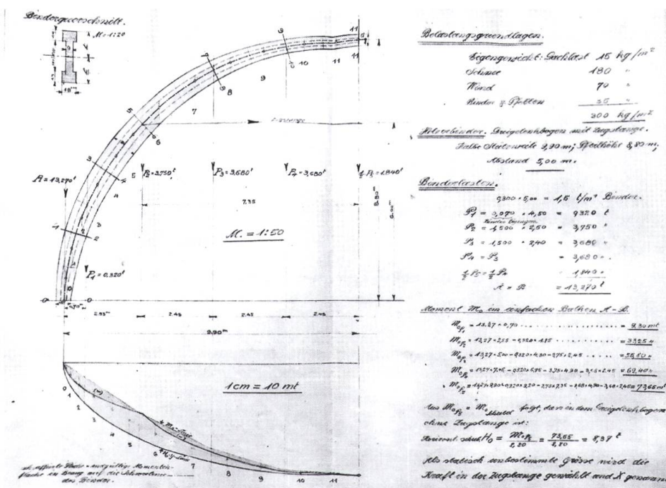
Abb. 12: Auszug aus der statischen Berechnung von Turner & Chopard vor dem Einbau der Zugstange 1917. (StAGR XX 179 E/1, S. 1–2)
