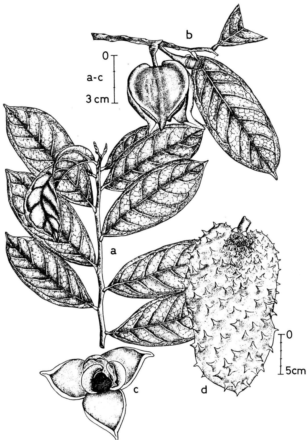
Fig. 2. — Annona muricata L. (Corossolier) a, rameau avec feuilles; b, rameau avec fleur et un jeune ovaire montrant, à son sommet, des étamines encore persistantes; c, une fleur montrant les pétales internes et l'androcée; d, fruit (Corossol).
