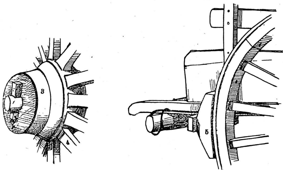
Fig. 92 e 93. — Parti del karettin : 1) la sa| . 2) al sivél . 3) la būsq|a . 4) i gavéj . 5) la tapéla .
