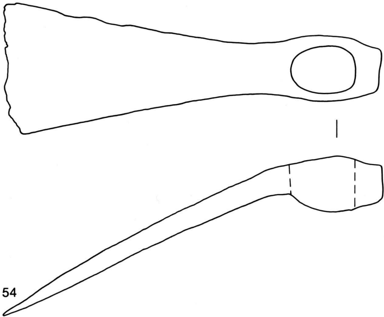
51-52: scies; 53-54: herminettes Ech.: 1:2
