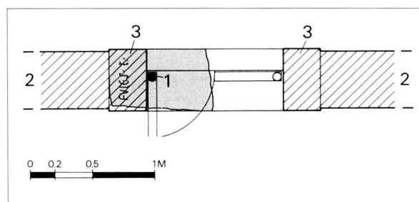
Fig. 2. Proposition de restitution schématique du seuil dans sa position originale. En gris, le fragment conservé; l'inscription se trouve ici sur une partie de la dalle encastrée dans la maçonnerie. 1: crapaudine. 2: mur. 3: chambranle. Dessin J.-P. Dal Bianco, MRA.
