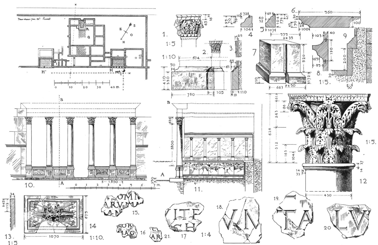
Abb. 26 Forum. Grabung 1913-1918 in Insula 40. Mutmasslicher Verwaltungsbau; Auszug aus dem Vorbericht von P. Schazmann. Tafel mit Architekturfragmenten und Rekonstruktionsvorschlag für die Säulenhalle H auf dem beigefügten Grundrissplan. Ohne Massstab.
