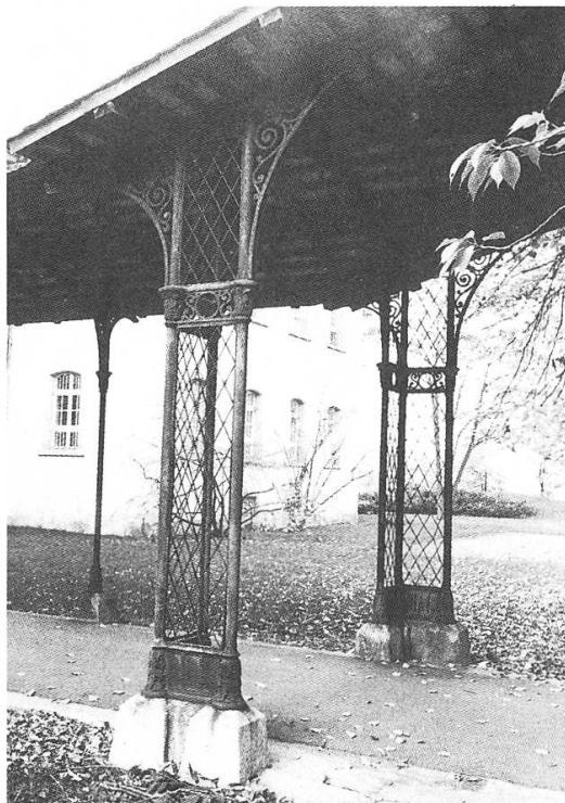
Abb. 18: Gusseisenkonstruktion in der Psychiatrischen Klinik Königsfelden.
