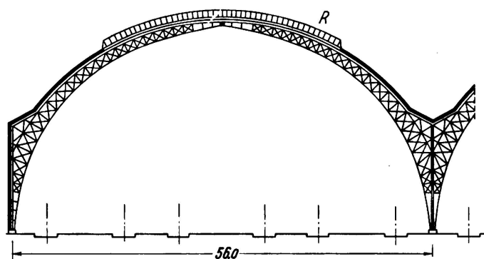
Fig. 1. Hauptbahnhof Frankfurt a. M. R Raupenoberlicht.
