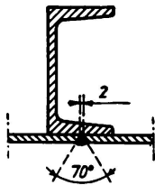
Fig. 5. Stonyschütze, Blechstoß auf \square -Eisenwischenträgern.
