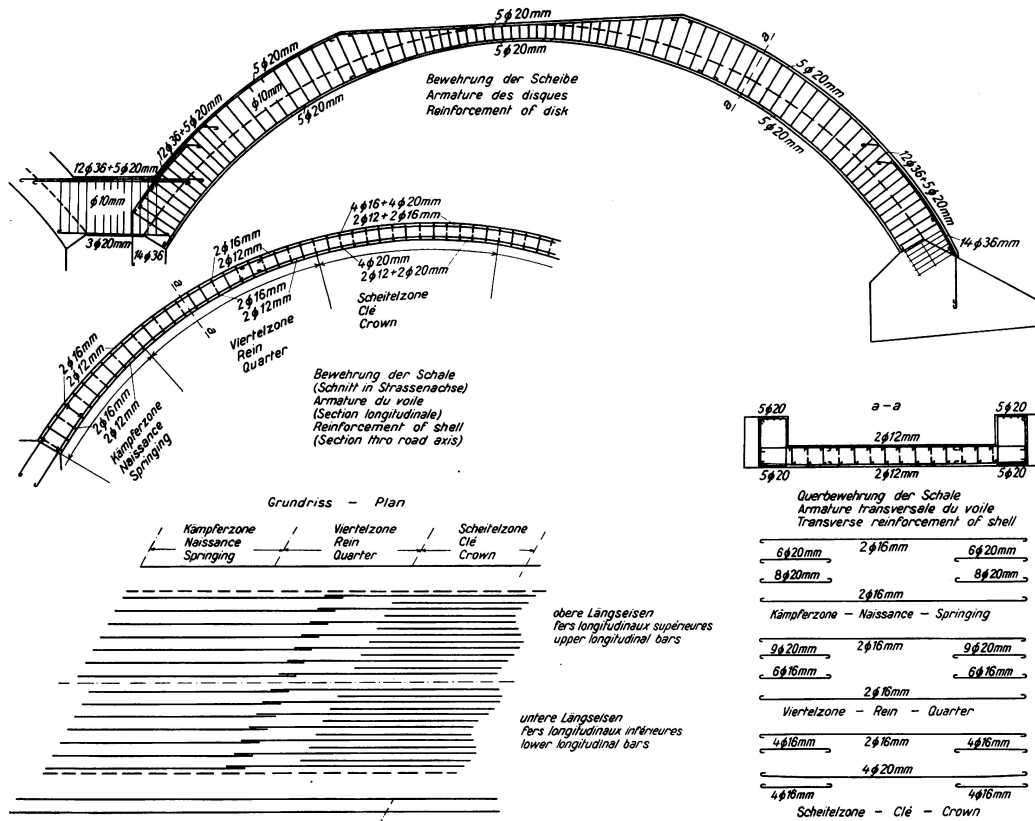
Fig. 2. Bewehrung der Gewölbe.
