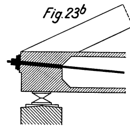
Fig. 22. Procédé de montage. Fig. 23. Pont à arc non rigide mis en tension préalable.
