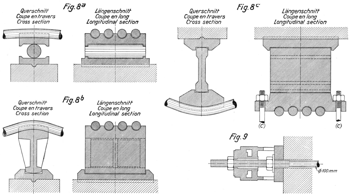
Fig. 8. 8a. Appui à rouleau pour la membrure de suspension. 8b. Appui à balancier pour la membrure de suspension. 8c. Appui à balancier pour la membrure de suspension avec balancier interchangeable.
