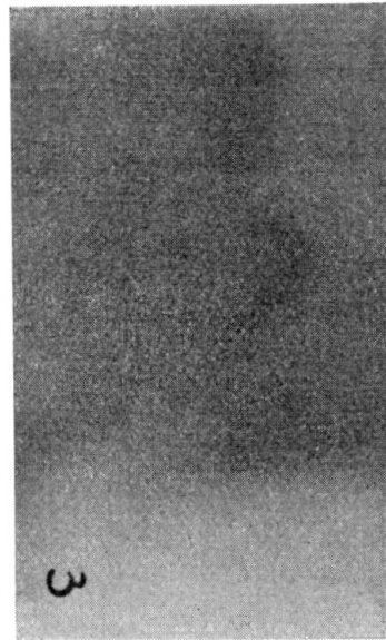
Spectre magnétique.
