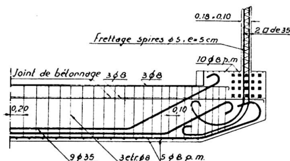
Fig. 5. Coupe transversale du tablier au droit d'une entretoise.
