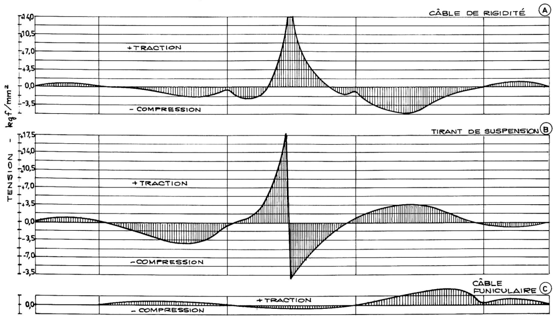
FIG.4 - LIGNES D'INFLUENCE DES TENSIONS
