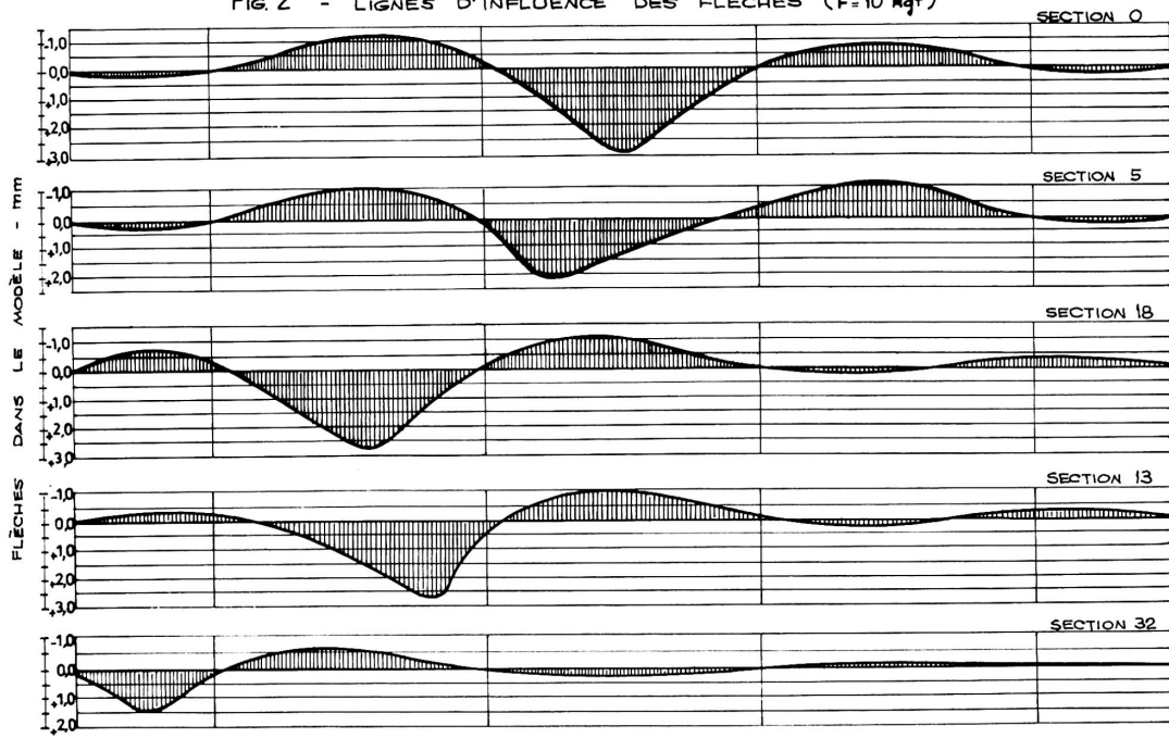
FIG. 2 - LIGNES D'INFLUENCE DES FLÈCHES (F=10 kgf)
