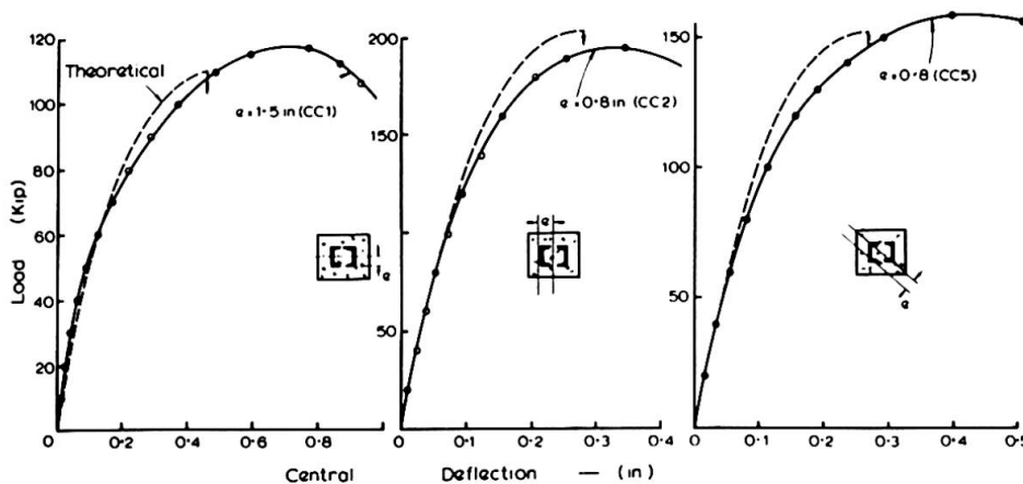
FIG. 11 BATTEN COLUMNS
