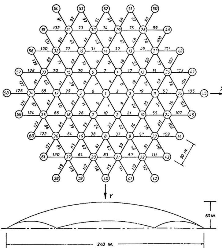
Bild 2: Fachwerkkuppel
