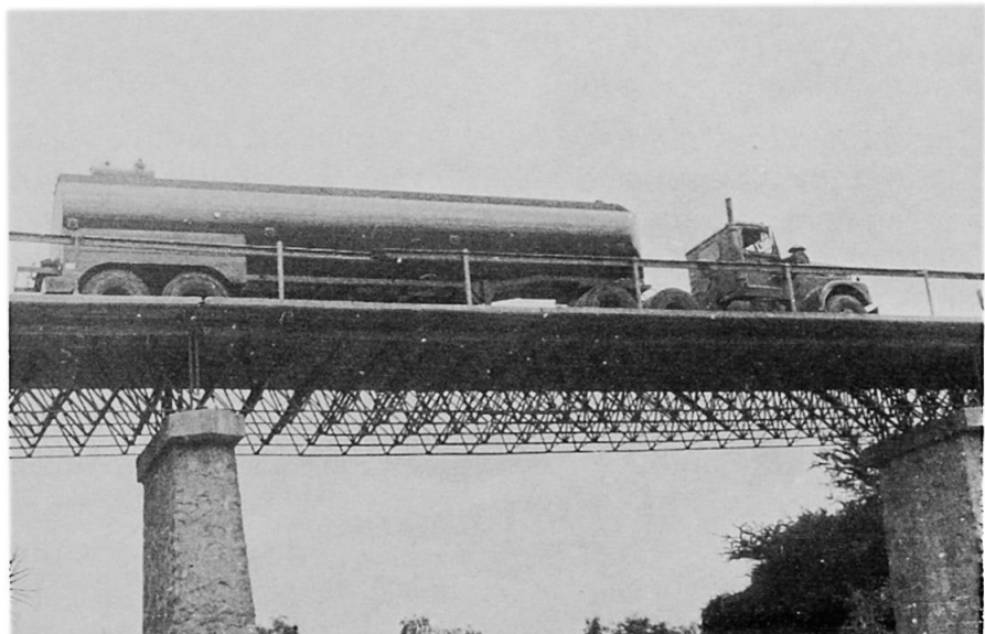
Fig. 7 Load Test
