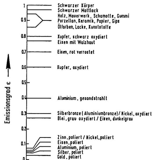
Fig. 3 Emissionsgrad einiger Materialien bei 10 µm [ 3 ]
