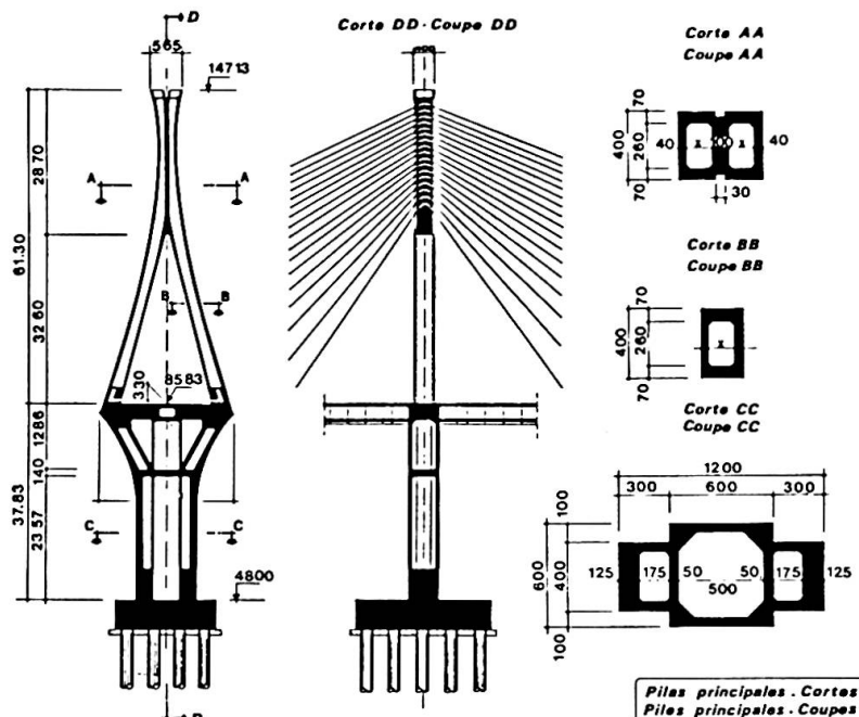
Figure 4 : Piles principales — Coupes
