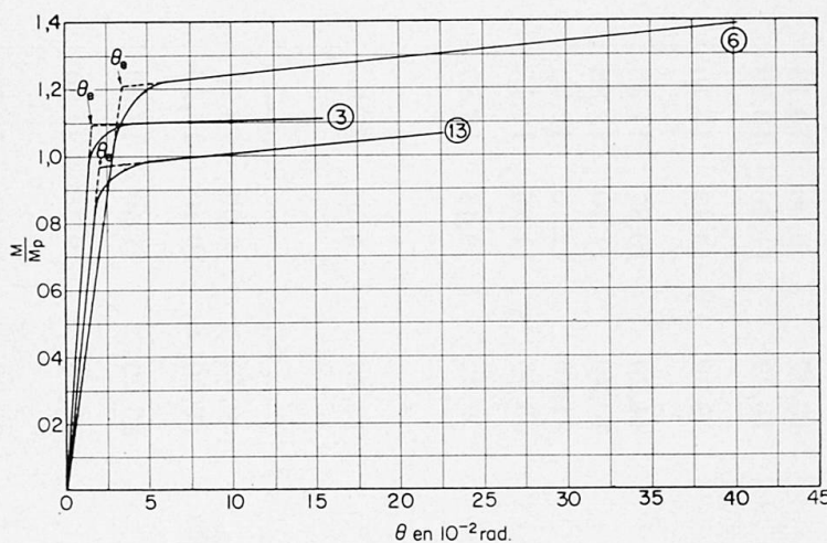
Fig. 8. Diagrammes moment-rotation.
