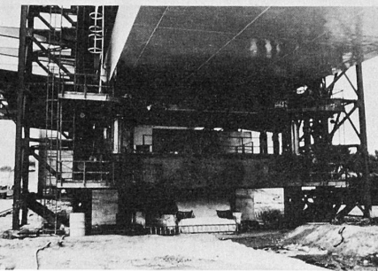
Plate-forme de levage du tablier
