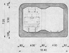
OUVRAGE FERROVIAIRE
