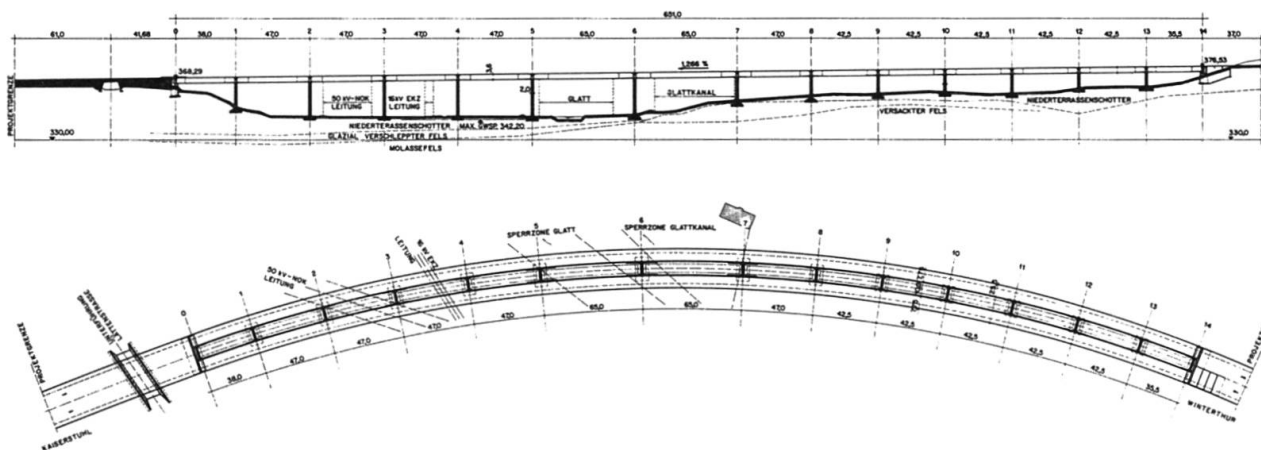
Längsschnitt
