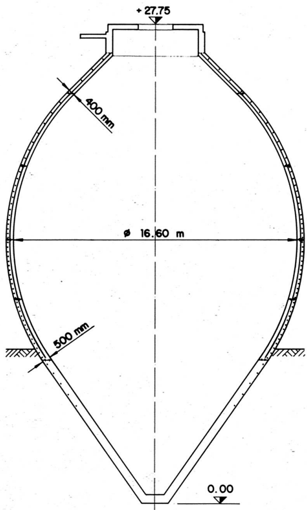
Bild 2: Schnitt durch einen der eiförmigen Behälter
