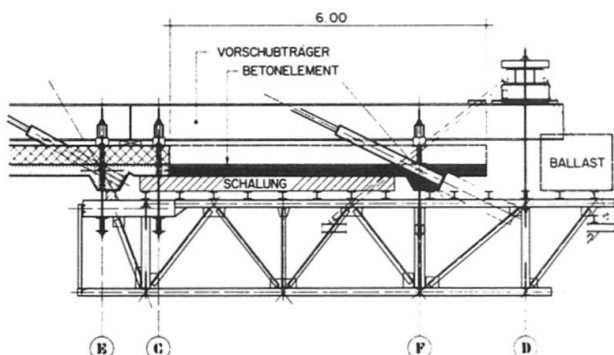
Bild 4. Vorbauwagen
