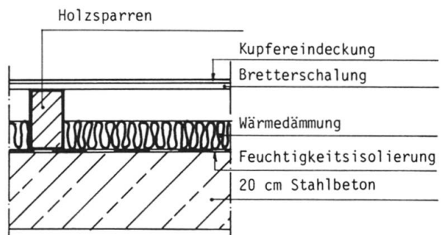
Fig. 1 Dachaufbau
