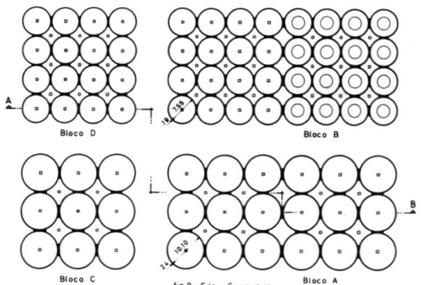
fig 9 - Silo - Geometria
