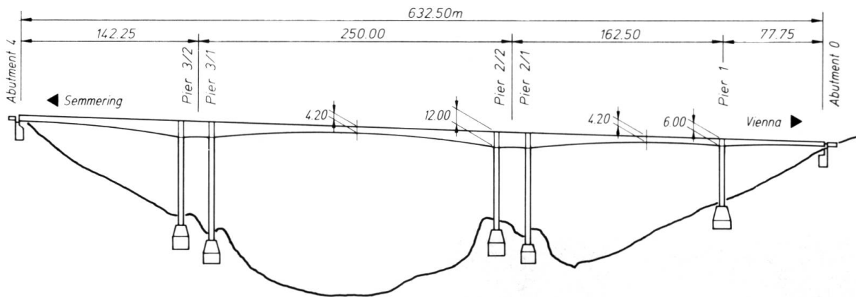
Fig. 4 Longitudinal section
