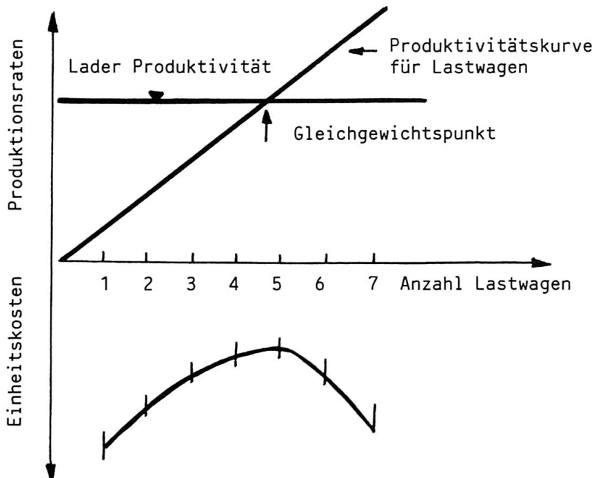
Figur 4. Produktivitäts- und Kostenkurven für ein deterministisches System
