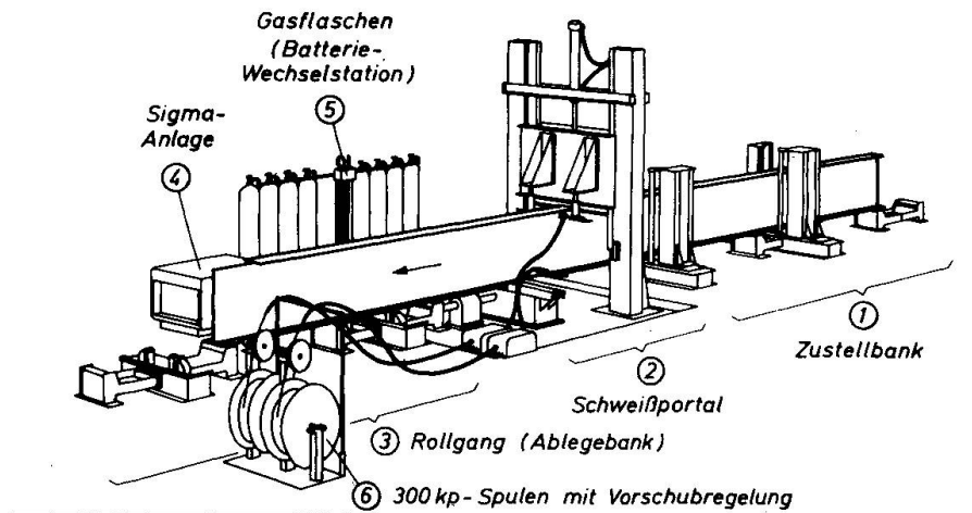
DONGES 4 - Naht - Schweißanlage UNIVERSITÄT BOCHUM KIB II
