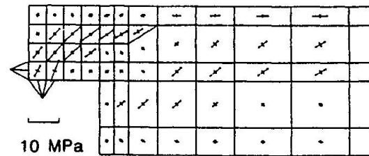
(d) Principal Concrete Stresses
