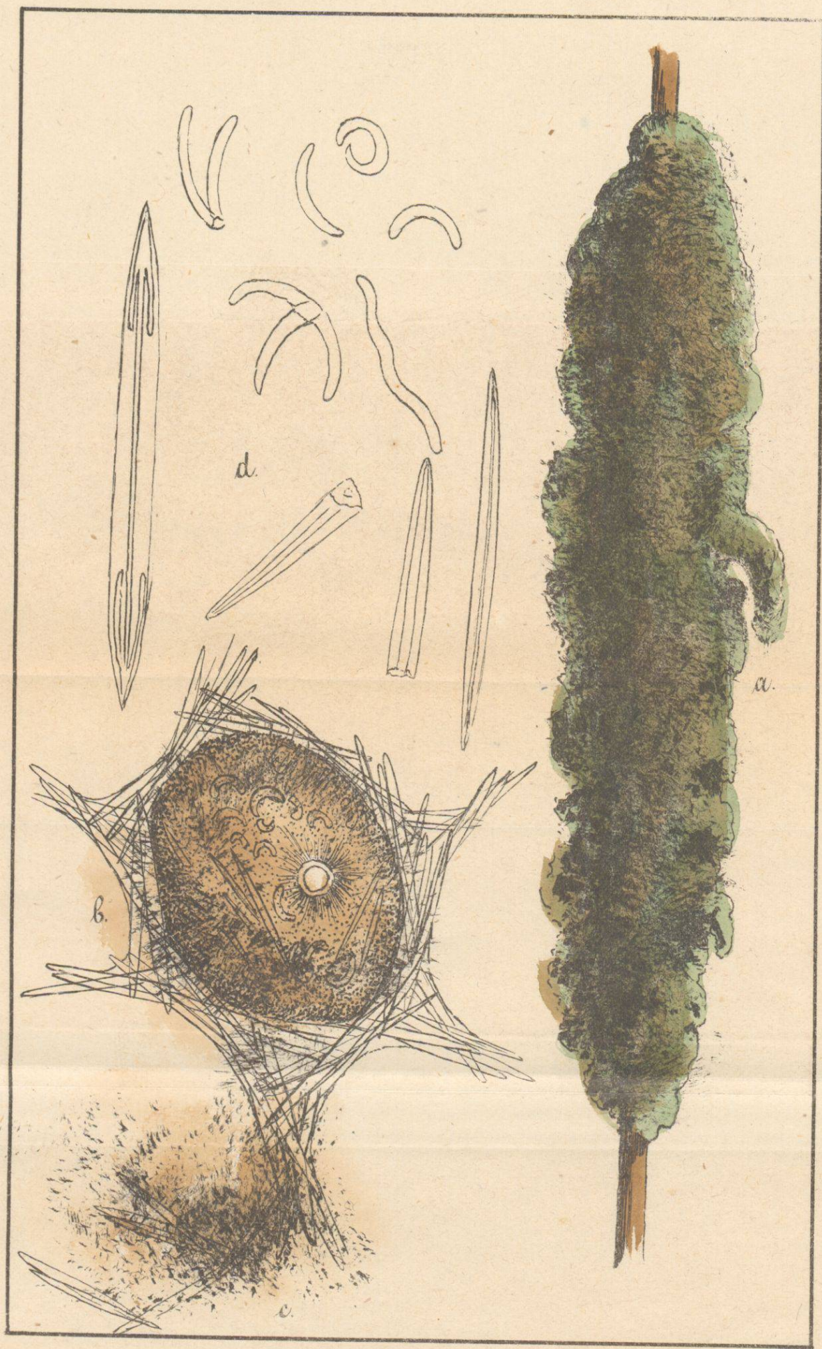
a. Éponge des roseaux. b. corps spongiaire dans sa cavité spiculaire. c. Sarcodé. d. Spicules de différentes formes.
