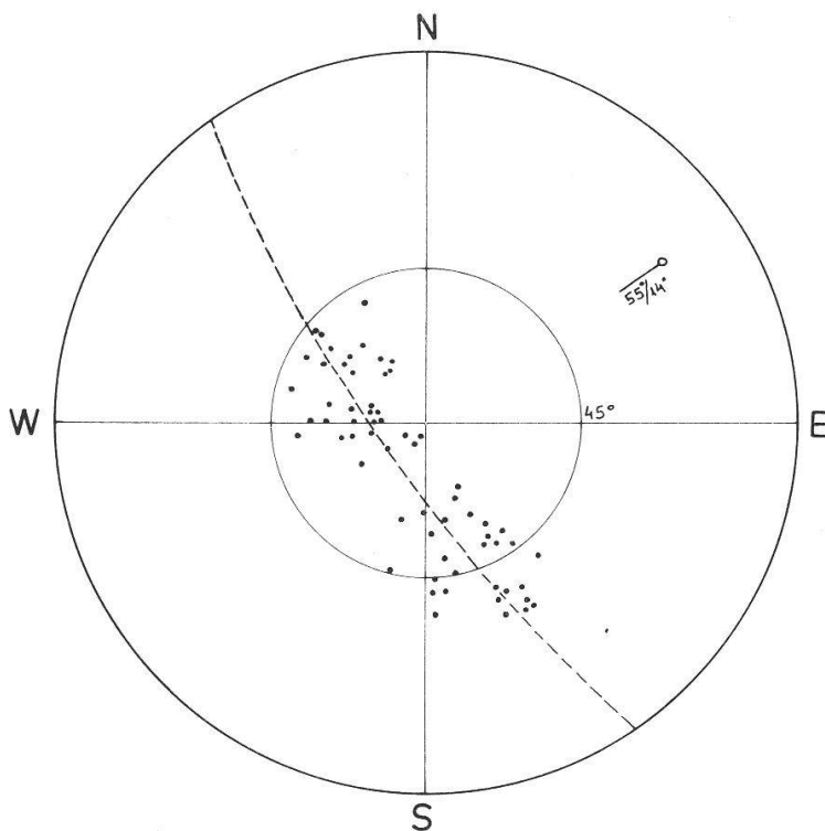
Fig. 4. Orientation de la voûte anticlinale dans la région de Saint-Blaise. Points = projection stéréographique (équiangle, hémisphère sup.) des couches sur les deux flancs de l'anticlinal ; ○— = projection stéréographique de l'axe de la voûte.
