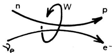
Fig. 4. — La désintégration du neutron considérée comme une interaction entre deux courants.
