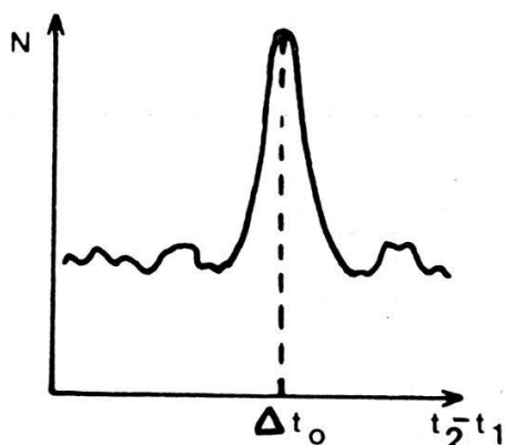
Fig. 1. — Principe d'une corrélation causale statistique. N : nombre de cas où P_2 se produit \Delta t après P_1 .
