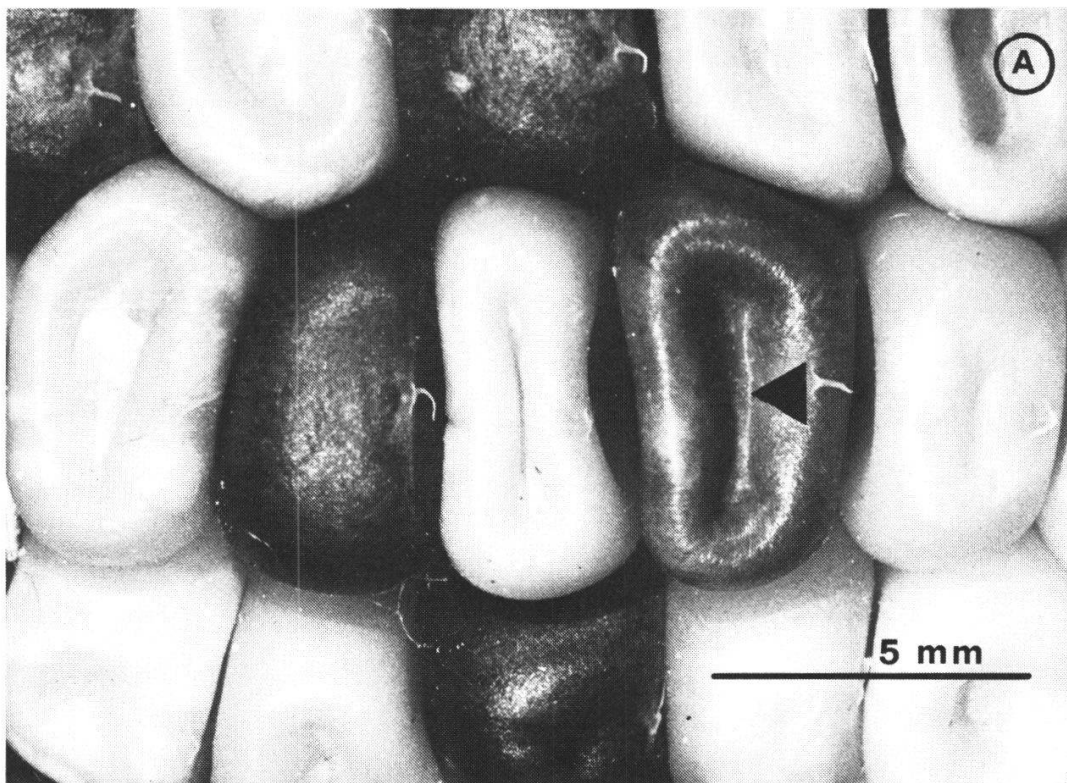
Figure 1A. – Détail d'un épi de maïs provenant du croisement entre un parent: sh_1 C^I / Sh_1 c et un parent: sh_1 c / sh_1 c . La morphologie de type «shrunk» (sous-production d'amidon) est visible sur les caryopses incolores, ceux-ci sont homozygotes pour le gène sh_1 , les hétérozygotes ( Sh_1 / sh_1 ) ont un aspect normal. Le caractère C^I allèle dominant détermine une absence de pigmentation (caryopses clairs), seul les caryopses c / c sont pigmentés. Les deux gènes sont portés par le chromosome 9, ils sont donc liés. L'application des lois de Mendel indique que l'on devrait avoir 50% de caryopses incolores-«shrunk» ( sh_1 c / sh_1 C^I ) et 50% de colorés-normaux ( sh_1 c / Sh_1 c ). La présence d'un caryopse ◀ coloré-«shrunk» indique un crossing-over entre les deux gènes.
