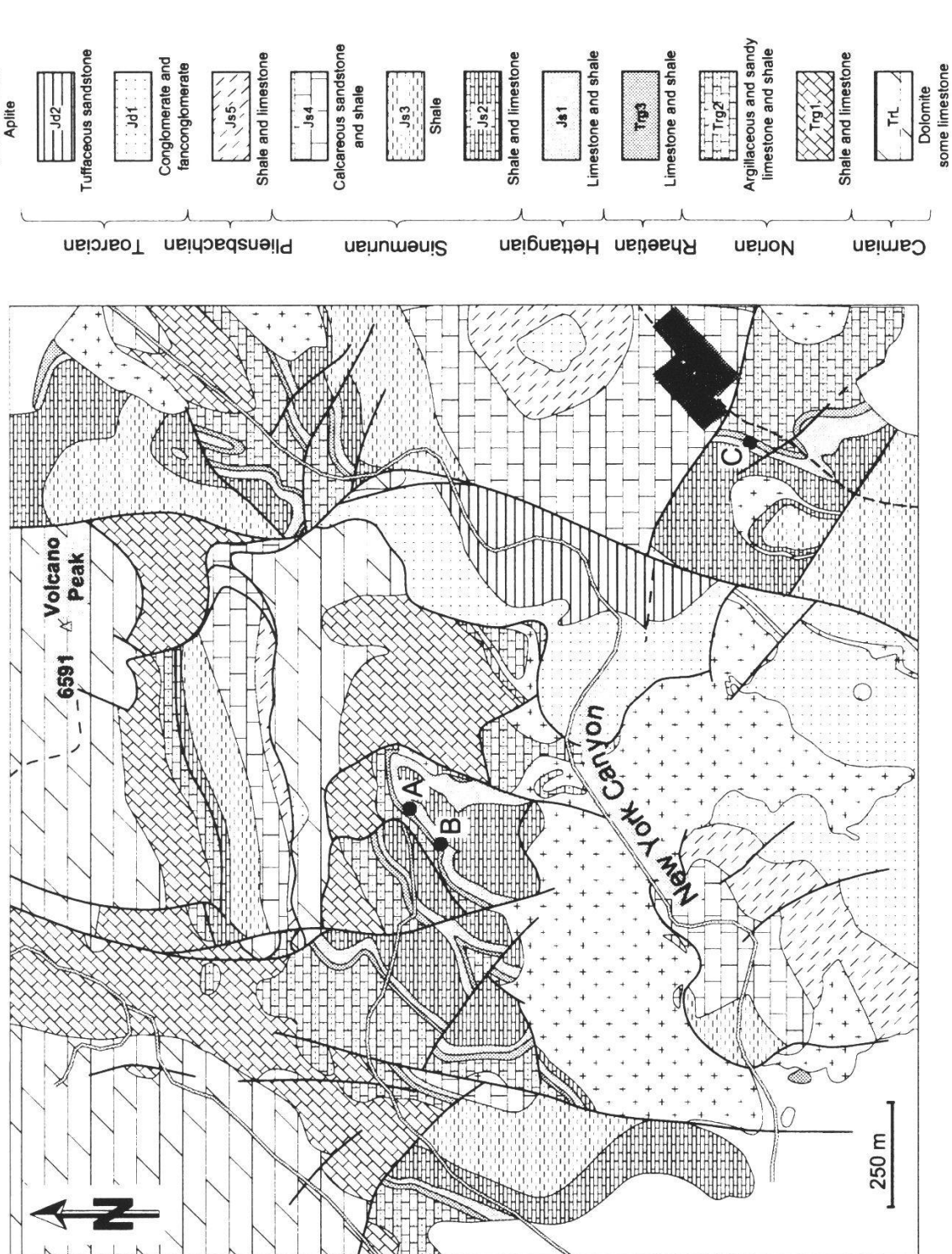
Figure 2.—Carte géologique du New York Canyon d'après FERGUSON et MULLER (1949) et localisation des coupes A à C dont une représentation synthétique est donnée dans la figure 3.
