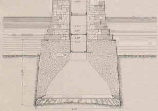
Caisson en béton pour la pile Fig 3 Section transversale 1:75
