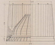
Fig 4 Elevation 1:75
