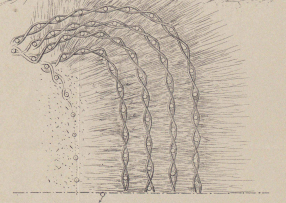
Fig. 3. Coupe en travers.
