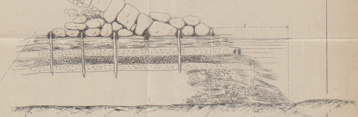
Fig. 3. Coupe en travers.
