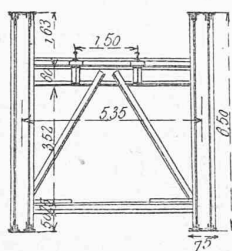
Fig. 12. — Coupe transversale du pont sur le Rhône, près Saint-Maurice.
