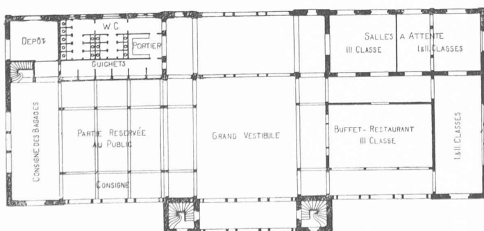
PLAN DU REZ-DE-CHAUSSÉE (1 cm. = 6 m.)
