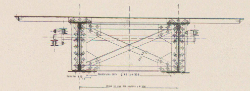
Coupe transversale suivant IJ
