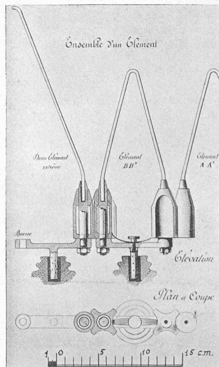
Fig. 1. — Détails de construction.
